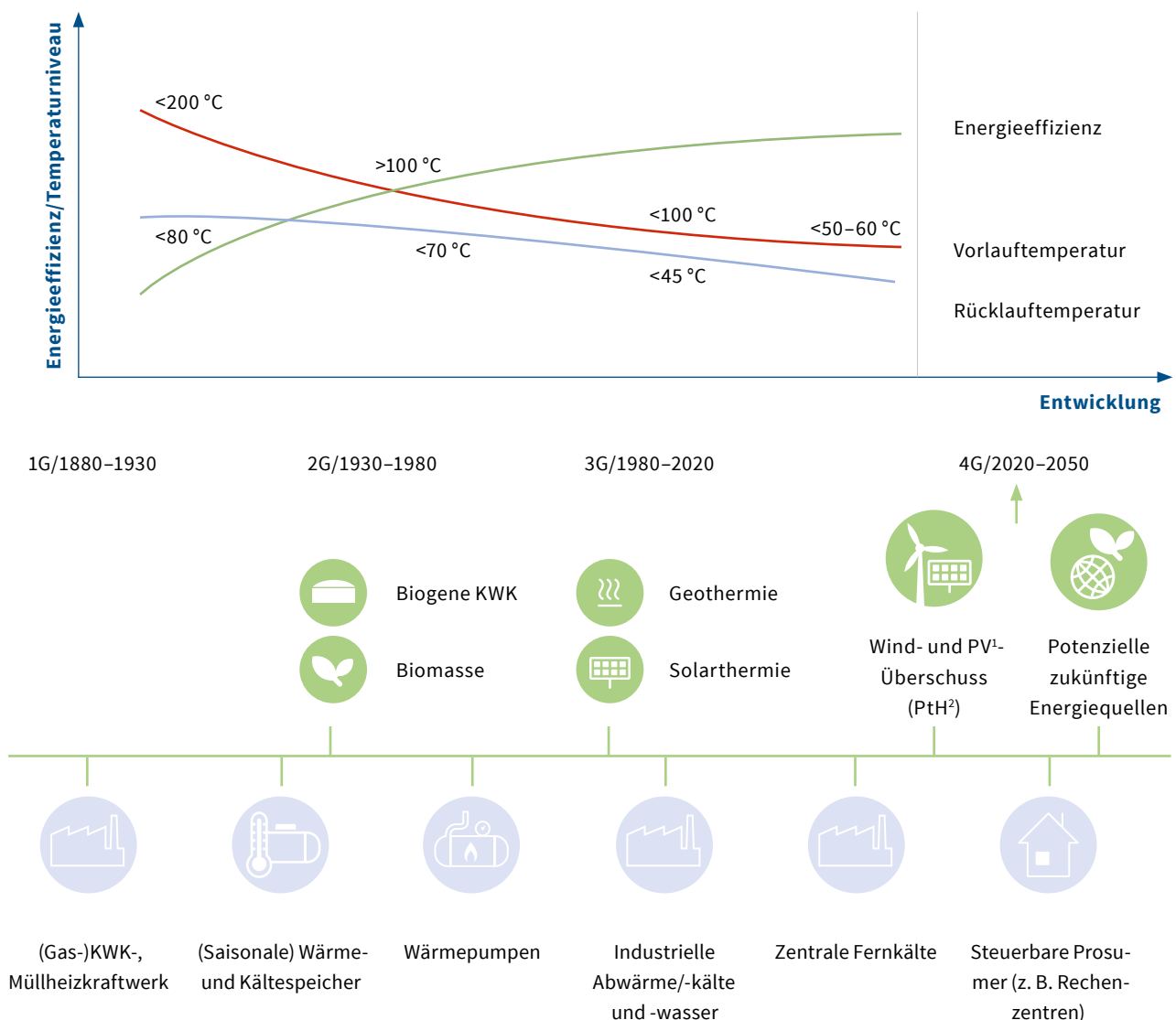
▼ Abb. 15: Vier Generationen der Fernwärme: Temperaturen, Energieeffizienz und mögliche Komponenten der künftigen bidirektionalen Fernwärme- und Fernkältenetze, Quellen: Lund et al. 2014 und Thorsen et al. 2018, eigene Darstellung
